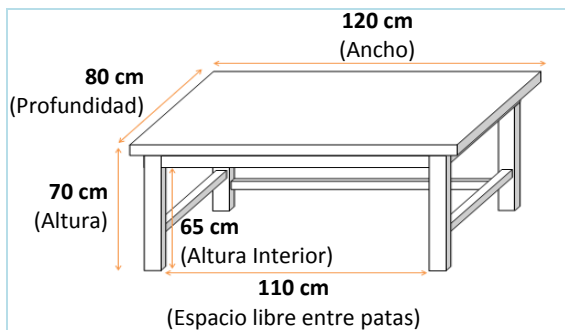
Figura 1: Esquema referencia para mesa alumnos.
