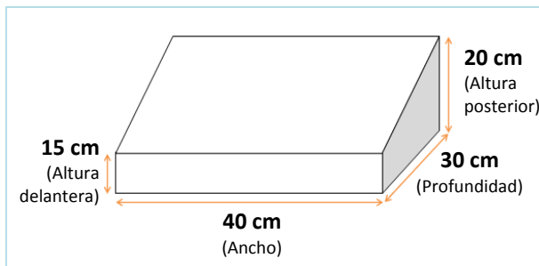
Figura 3: Esquema de referencia para reposapiés.
