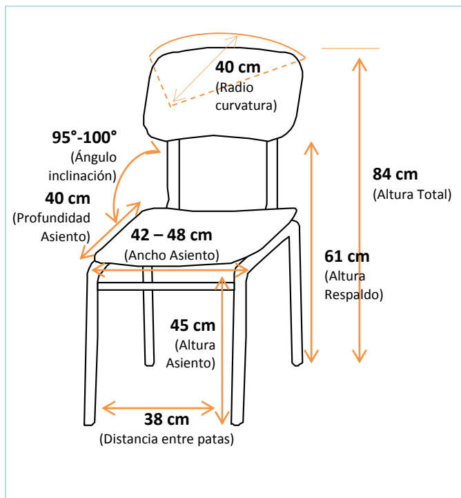
Figura 2: Esquema de referencia para silla de alumnos.
